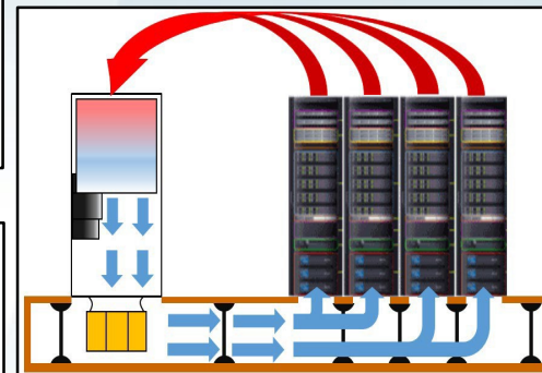
Подача нисходящего потока (вентиляторный радиатор)
