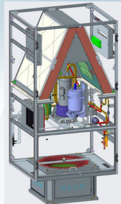
Вентилятор с нисходящим потоком воздуха
